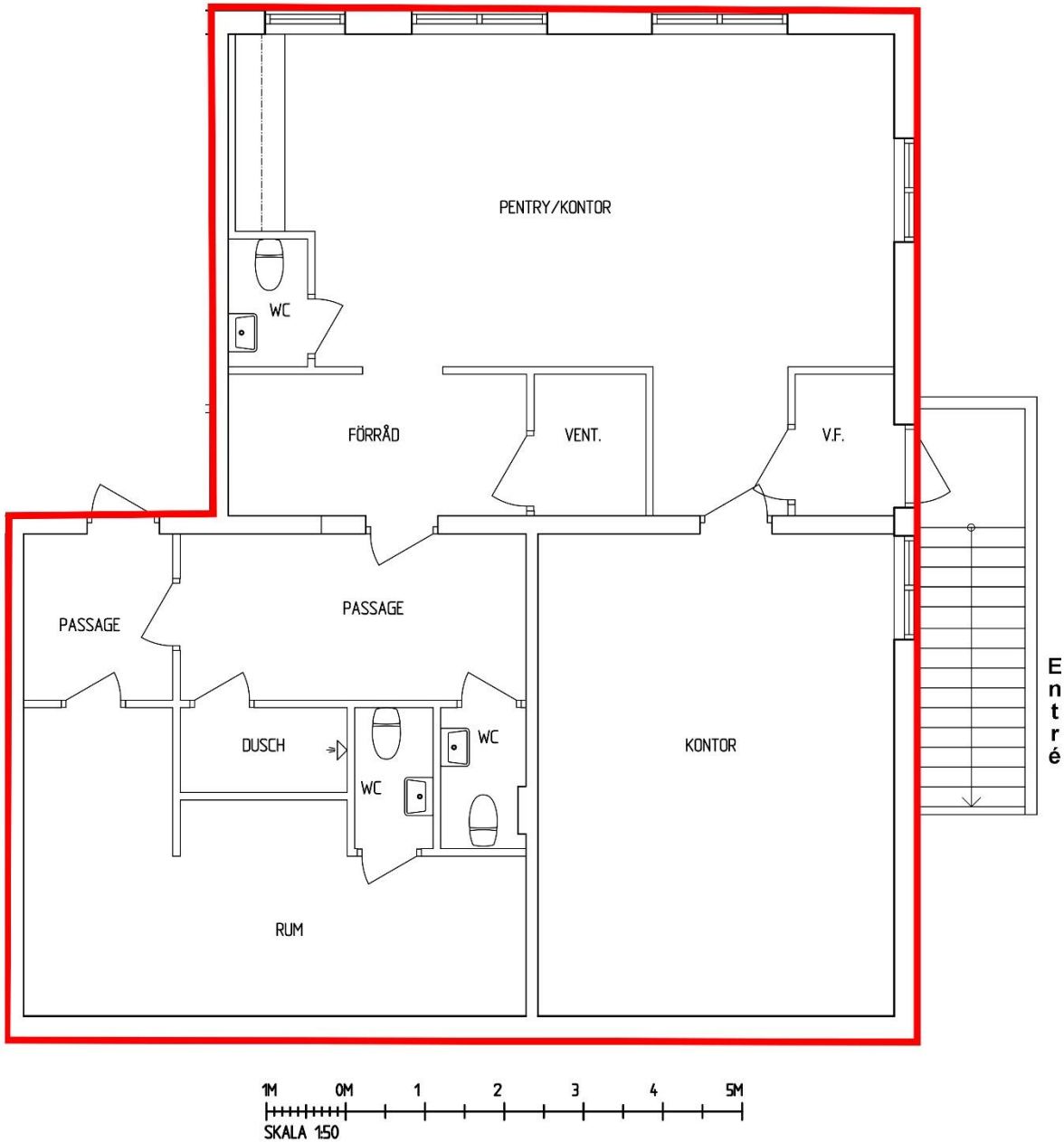
PLAN 1 - KÄLLARPLAN
