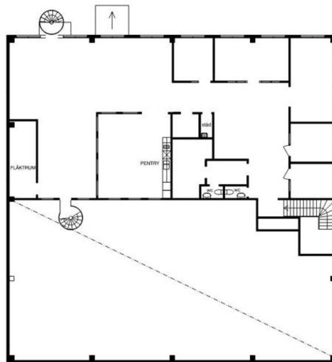
PLAN1 1:200
