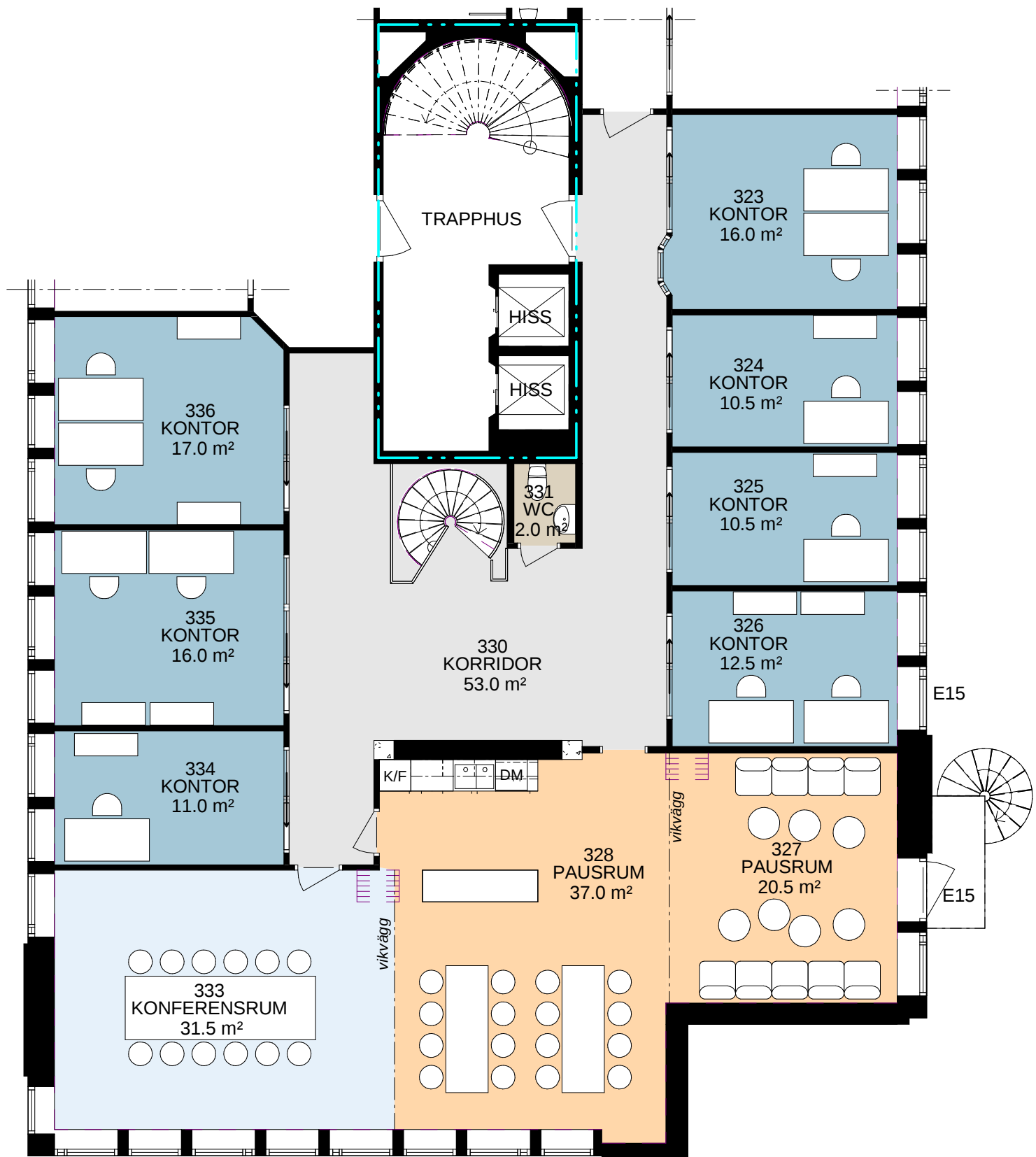
PLAN 5 (VÅN 3)
