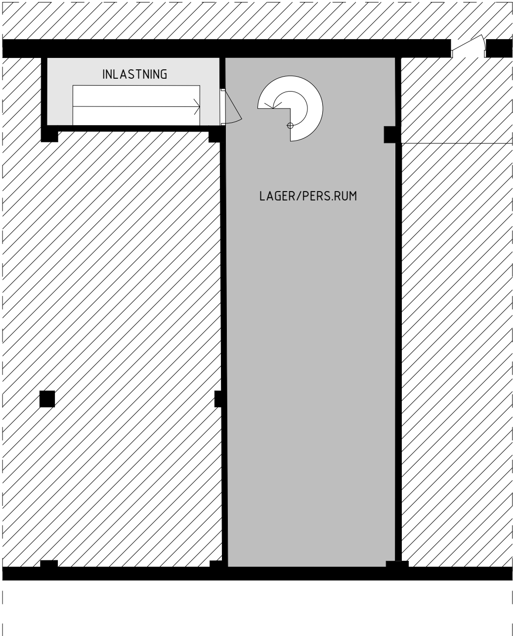
KÄLLARPLAN
