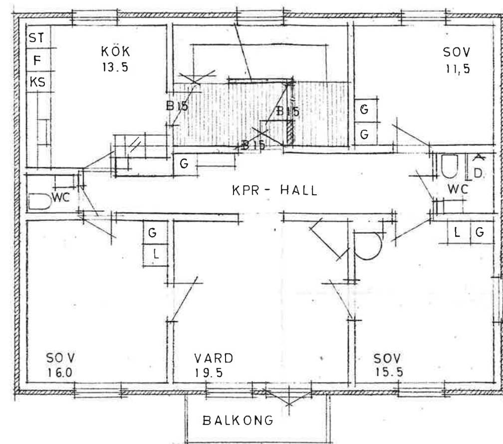
VÅNINGSPLAN 1 TR
