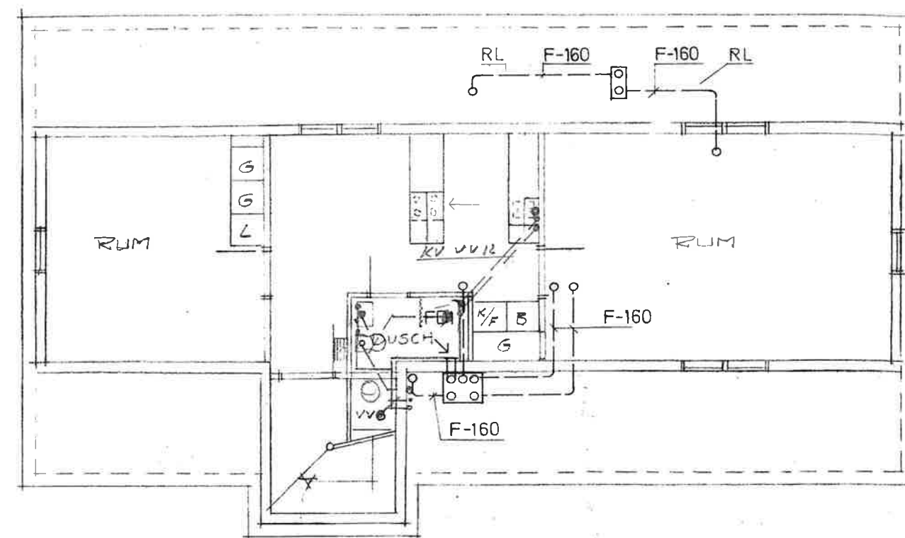
VINDPLAN
