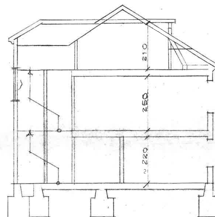
SEKTION
