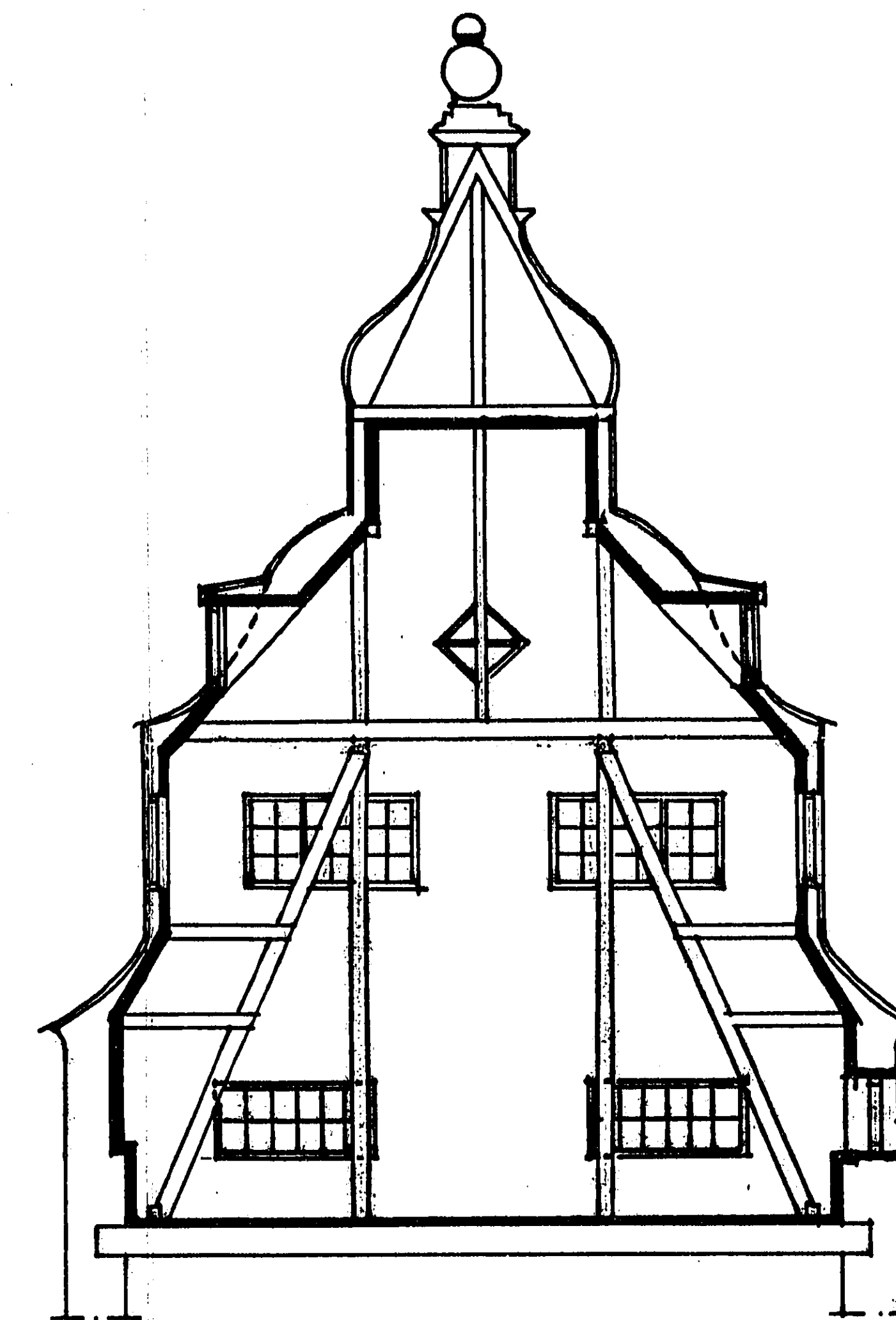
SEKTION B-B
