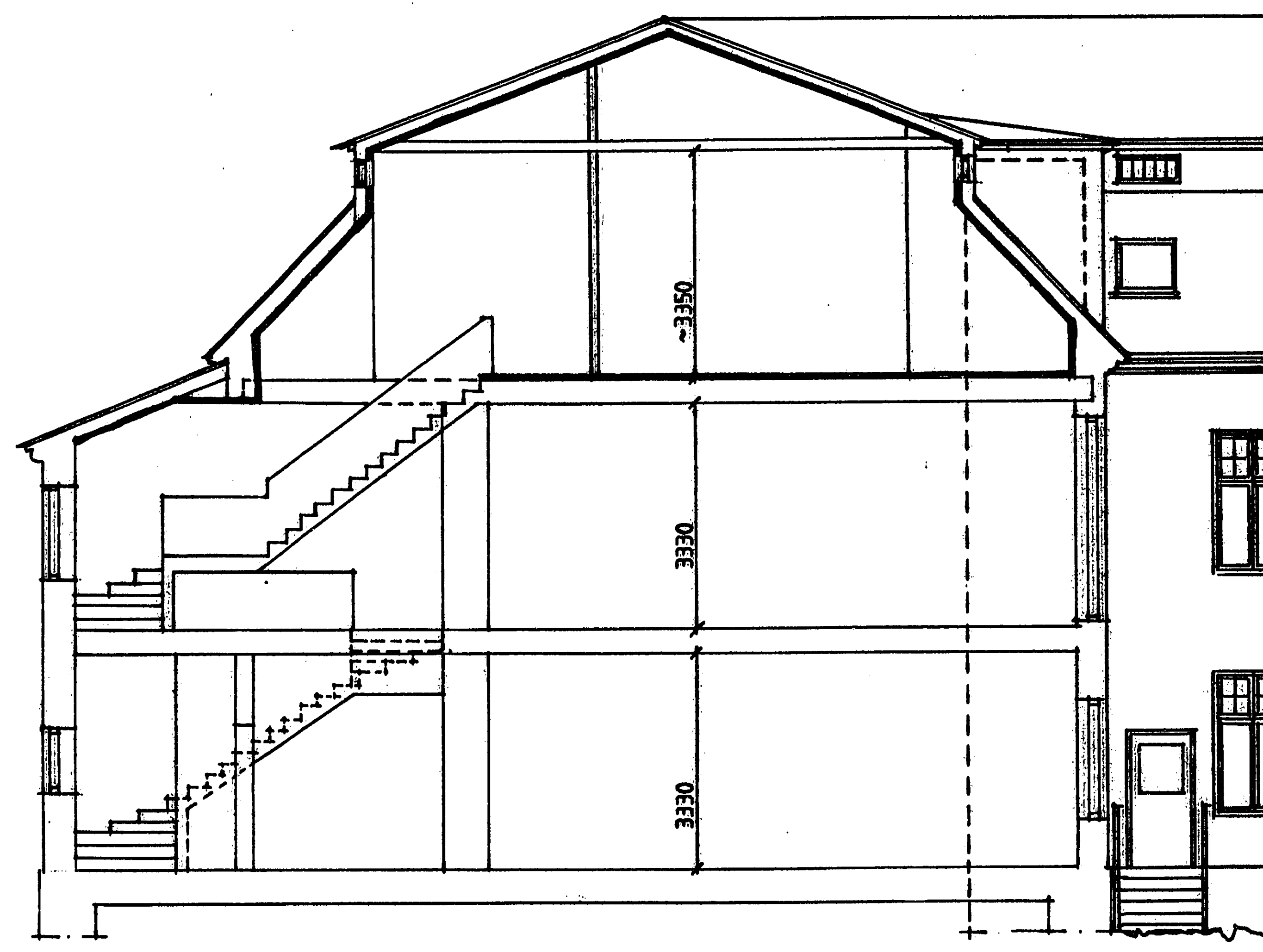
SEKTION A-A
