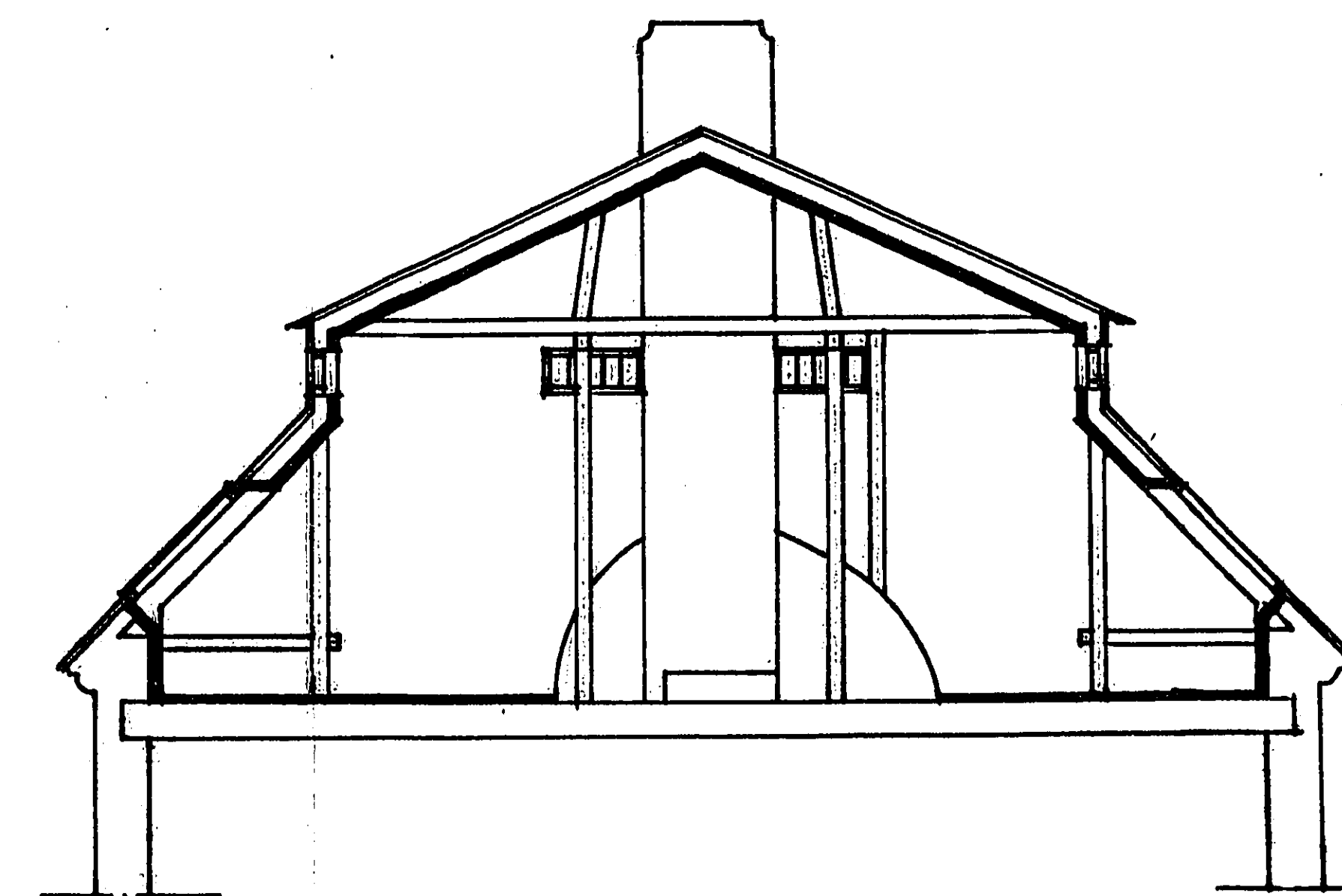
SEKTION C-C
