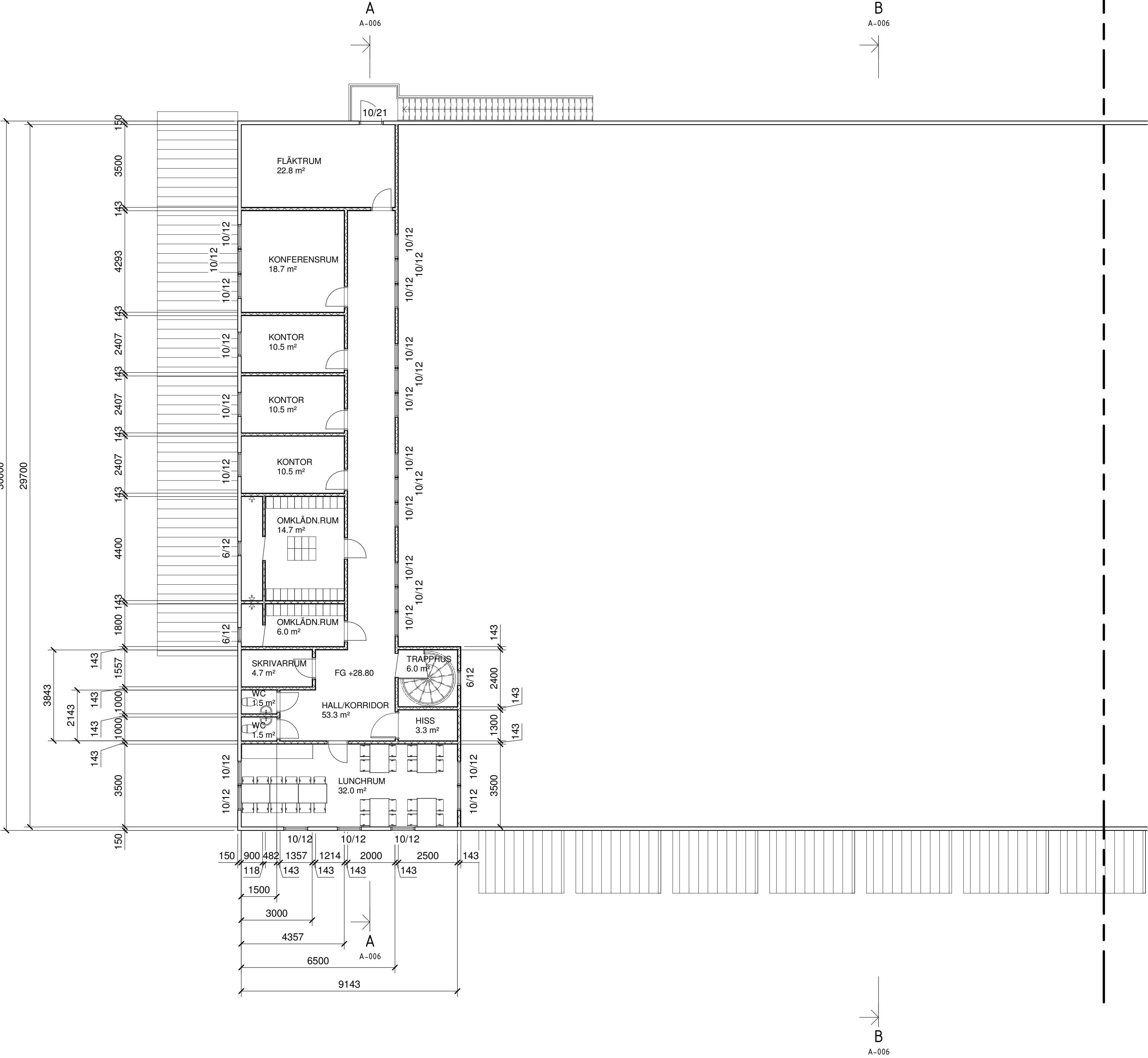
MÄTTSATT PLAN, PLAN 1, DEL 1 1 : 100
