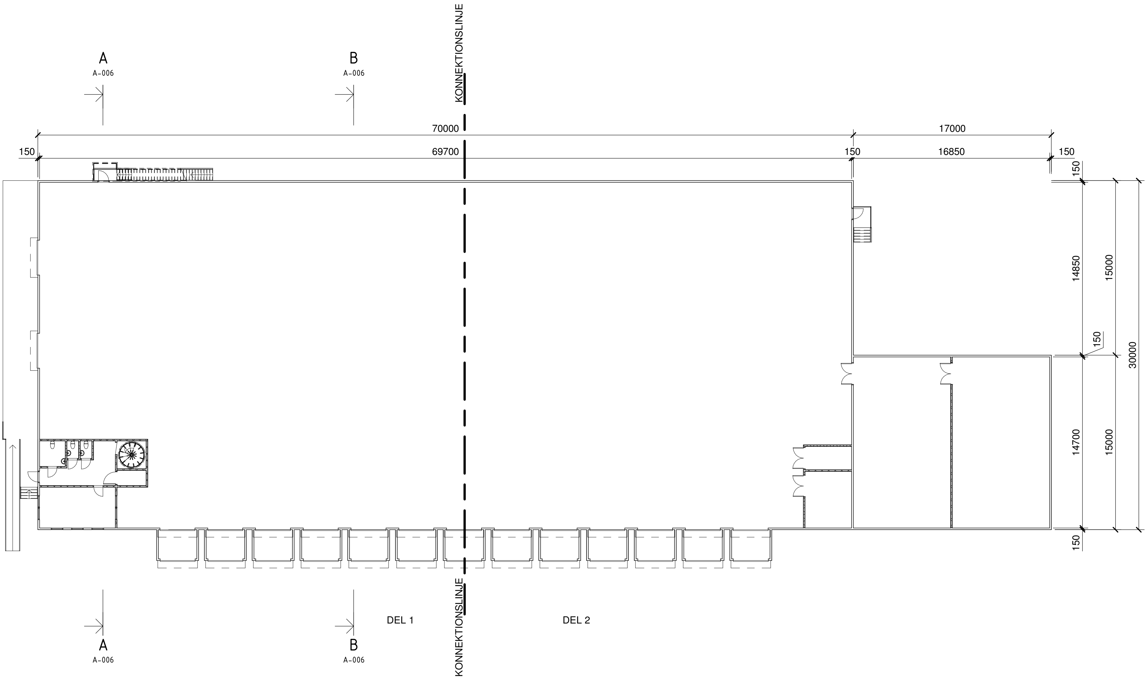
MÄTTSATT PLAN, PLAN BV 1 : 200
