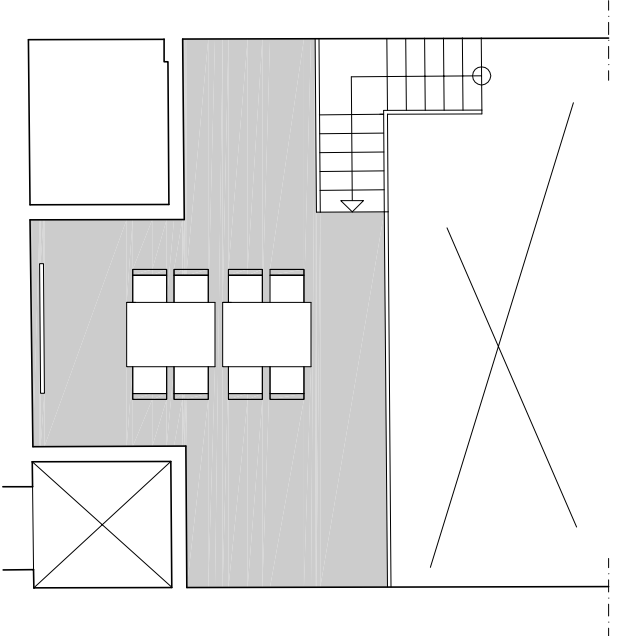
PLAN ENTRESOLPLAN
